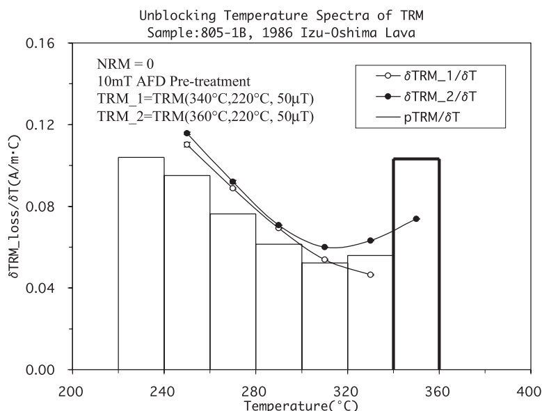
図 2 PSD-like 粒子群の高温粒子群から低温粒子群への影響を示す。試料を強磁性鉱物が化学変化する以下の温度で 2 回着磁した。第 1 回目の TRM_1 (340°C, 220°C, 50 μT) は、上限温度 340°C から下限温度 220°C まで 50 μT の定常磁場で自然冷却を、220°C より室温まで無磁場空間に強制冷却を行った過程で獲得した。TRM_2 (360°C, 220°C, 50 μT) は上限温度を 360°C に上げた点のみが TRM_1 と異なる。それぞれの TRM について段階消磁を実施し、その unblocking 温度 \delta TRM を調べた。TRM_1 と TRM_2 との unblocking 温度分布の違いは、高い blocking 温度 ( T_b : 340°C ~ 360°C) 粒子集団から低い T_b (220°C ~ 340°C) 粒子集団の unblocking 温度分布への影響を反映する。高温粒子集団の擾乱はその直下温度範囲 (300°C ~ 340°C) 粒子集団に留まり、より低い温度へはほとんど影響を及ぼさない。参考のため pTRM の分布も示した。
